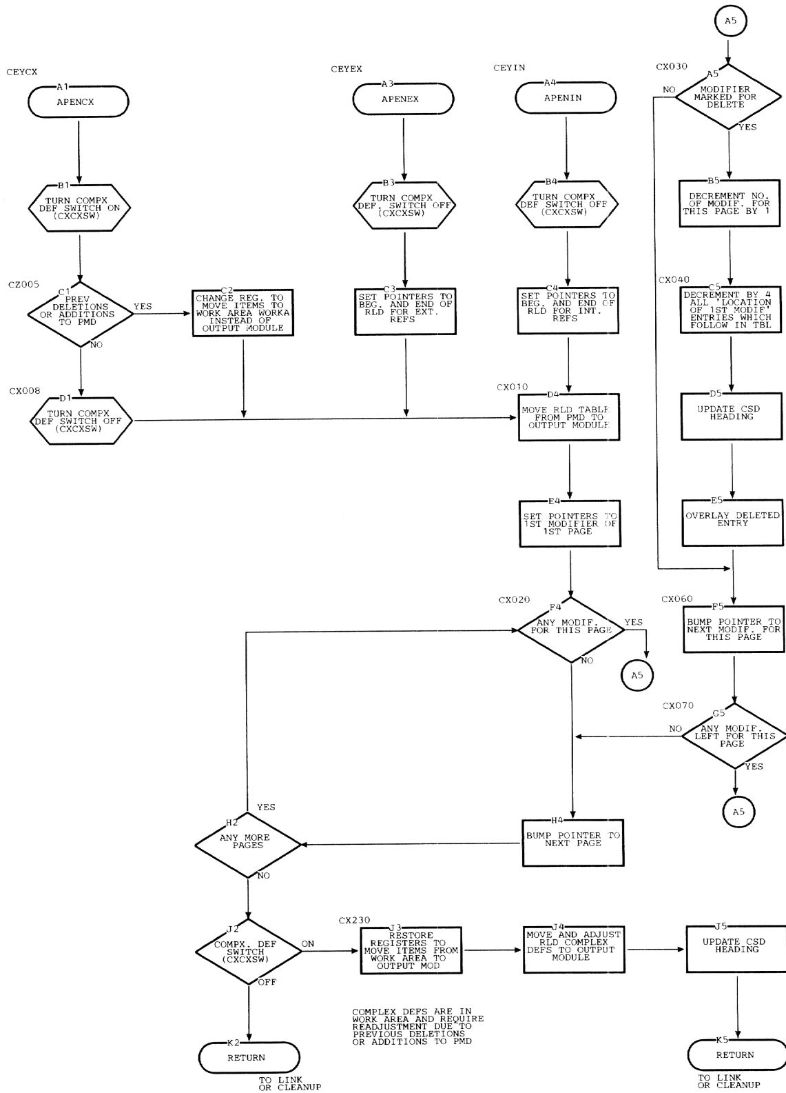
Chart AM. APENCX, APENEX, and APENIN
